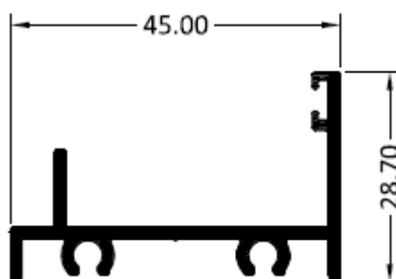
5057 CIERRE INFERIOR
