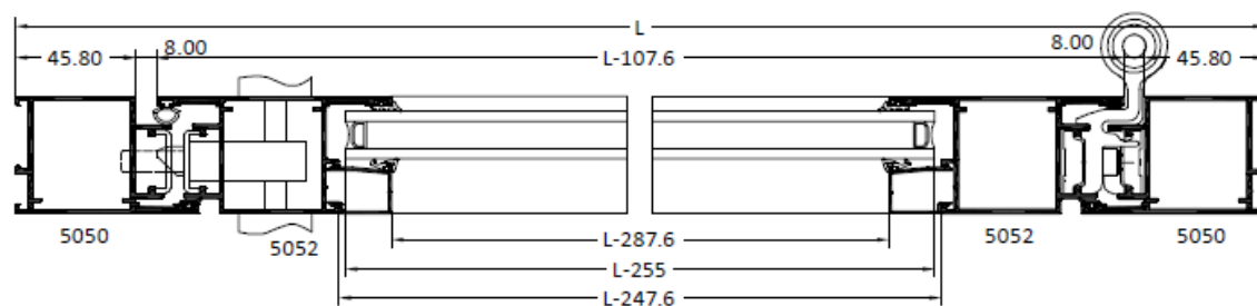
SECCIÓN HORIZONTAL A-A'
