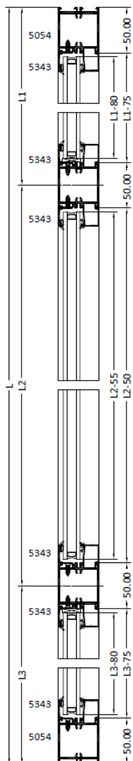
SECCIÓN B-B?
