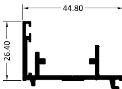
5057 SUPLEMENTO MARCO
