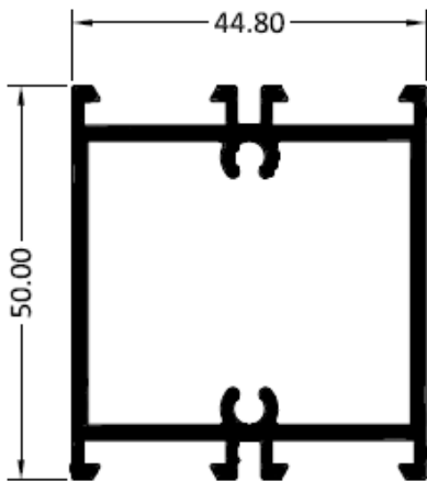
5054 TRAVESAÑO DE 50mm
