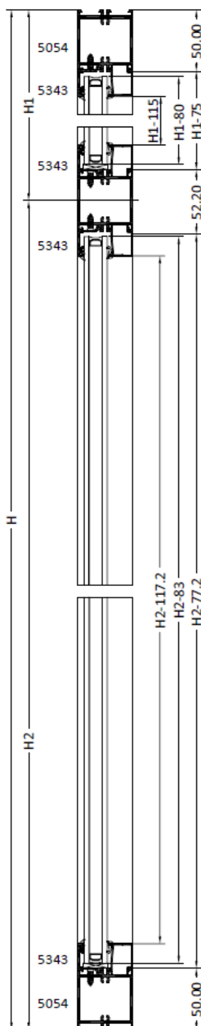
SECCIÓN D-D?
