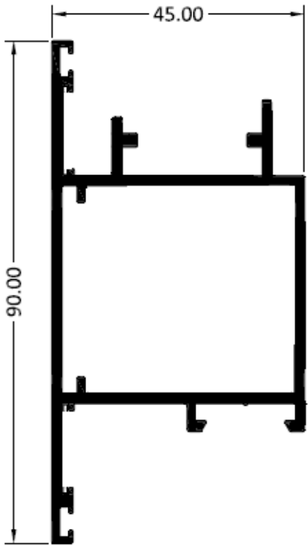
5052 HOJA APERTURA INTERIOR
