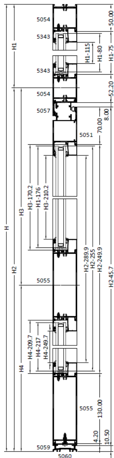
SECCIÓN C-C?
