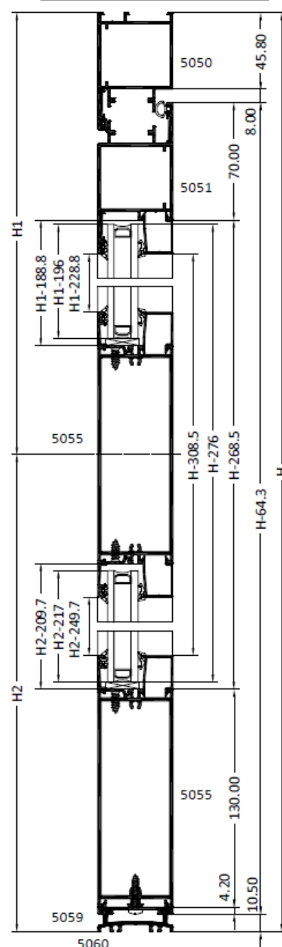
SECCIÓN VERTICAL B-B'
