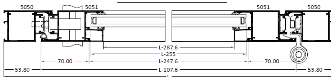
SECCIÓN HORIZONTAL A-A'
