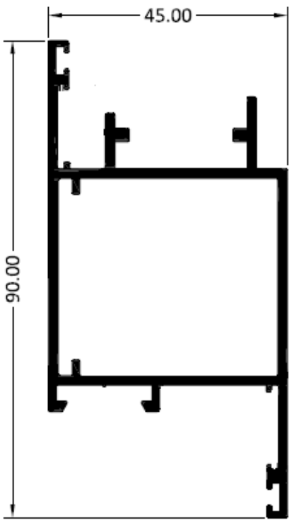
5051 HOJA APERTURA INTERIOR
