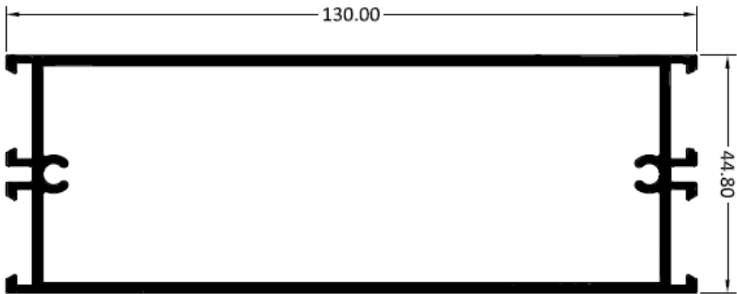
5055 TRAVESAÑO DE 130 mm
