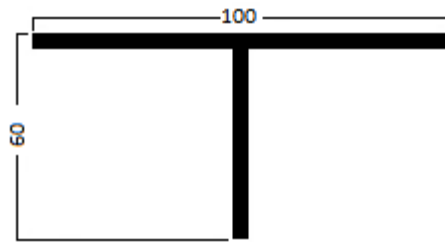
13149 PERFIL T DE 100x60x2mm
