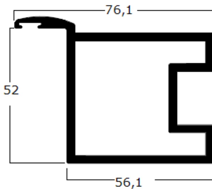
9683 MARCO PORTALES 50 mm C/ BATIENTE
