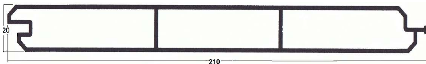
CMD6222 CHAPA TUBULAR 200x20
