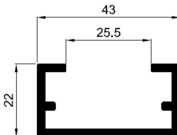
8104 LAMA PARASOL 120mm
