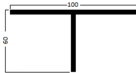
13149 PERFIL T DE 100x60x2mm
