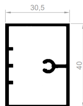
PERFIL REFUERZO HORIZONTAL
