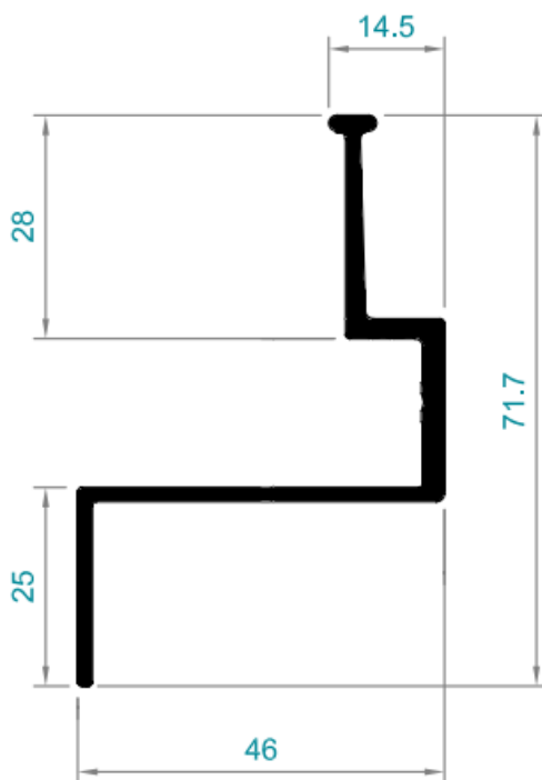
E15453 FIJACION MACHO FACHADAS
