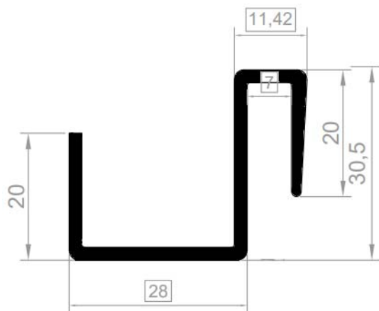
PERFIL HEMBRA FACHADAS
