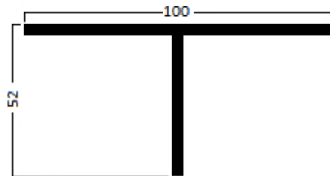
42024 PERFIL T DE 100x52x2mm
