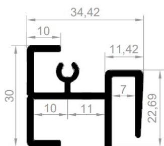
PERFIL RIGIDAZOR
