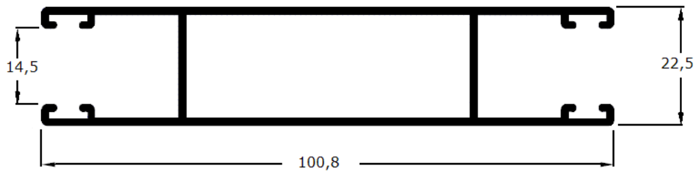
2806 GUIA MONOBLOCK DOBLE 108 mm
