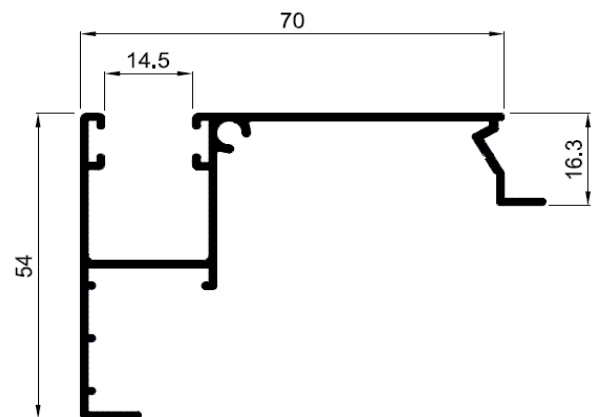
1037 GUIA MONOBLOCK DE 70 mm
