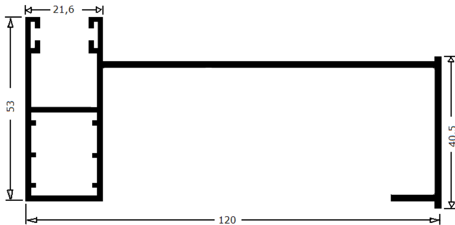
2937 GUIA COMPACTO REC. EMBUTIR 120 mm
